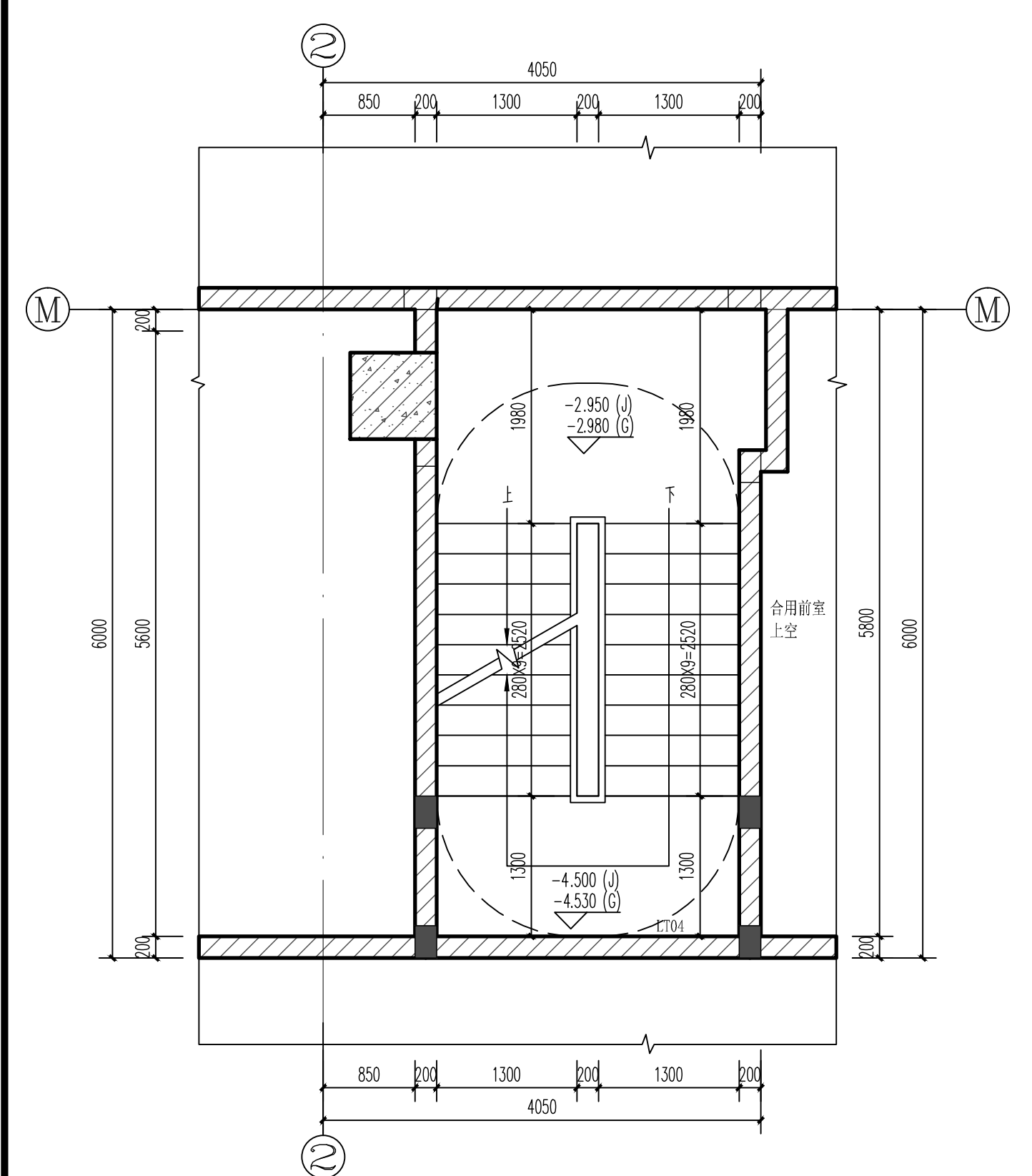
比例 LT04 -2.950m标高平面 1:50
