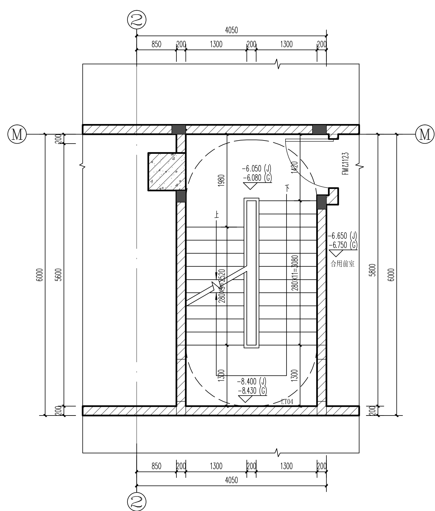
比例 LT04 地下一层平面 1:50
