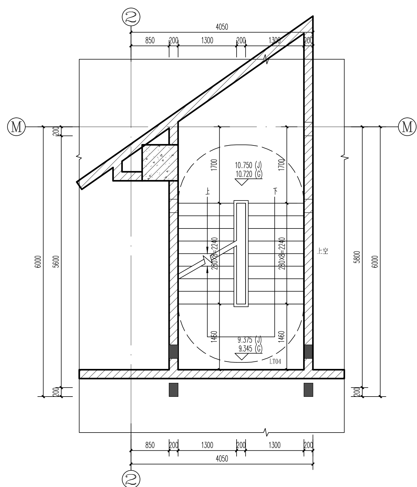
比例 LT04 10.750标高平面 1:50
