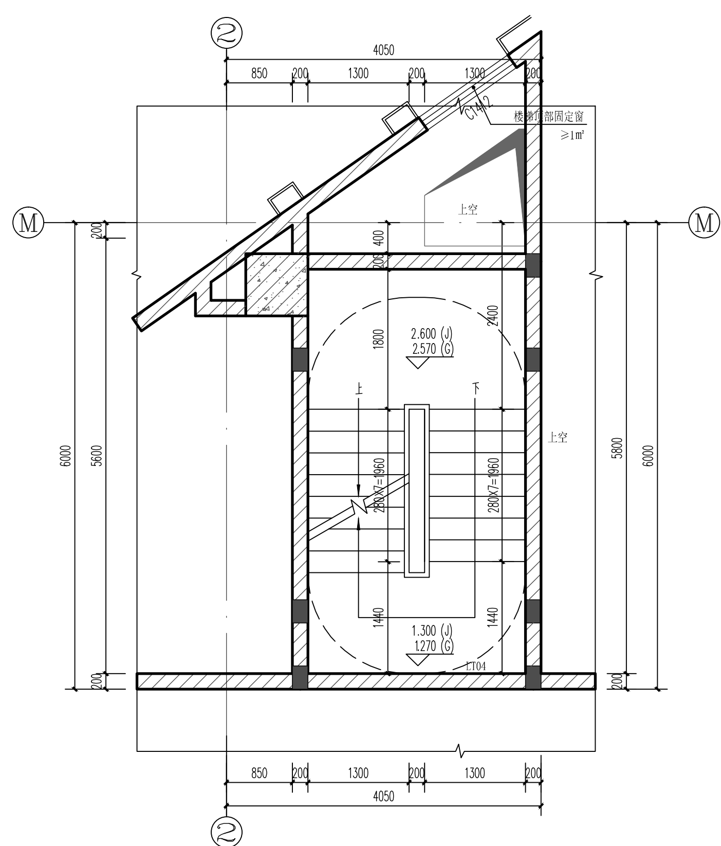
比例 LT04 2.600m标高平面 1:50
