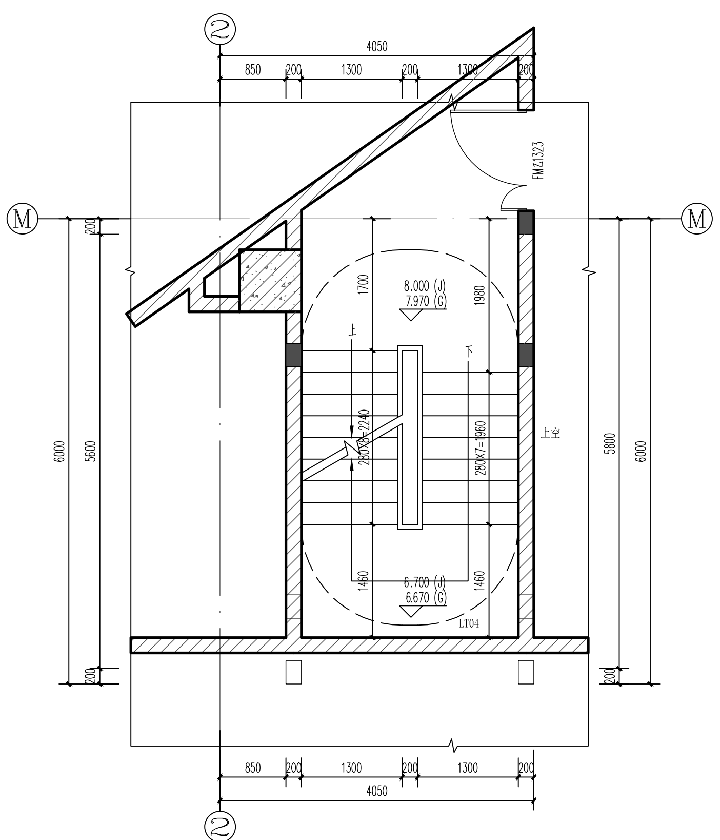
比例 LT04 5.400m标高平面 比例 LT04 二层平面 1:50 1:50
