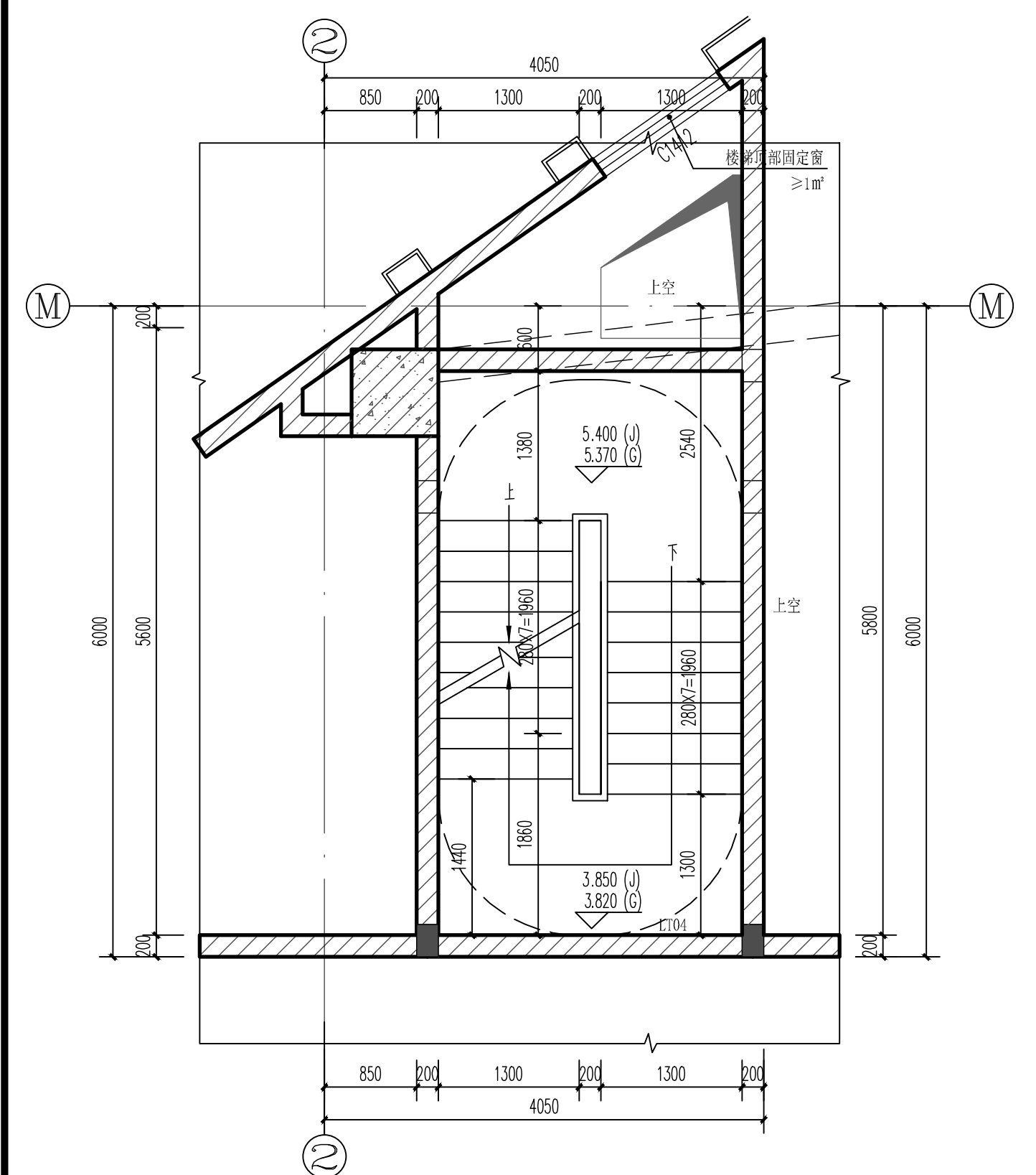
比例 LT04 5.400m标高平面 1:50
