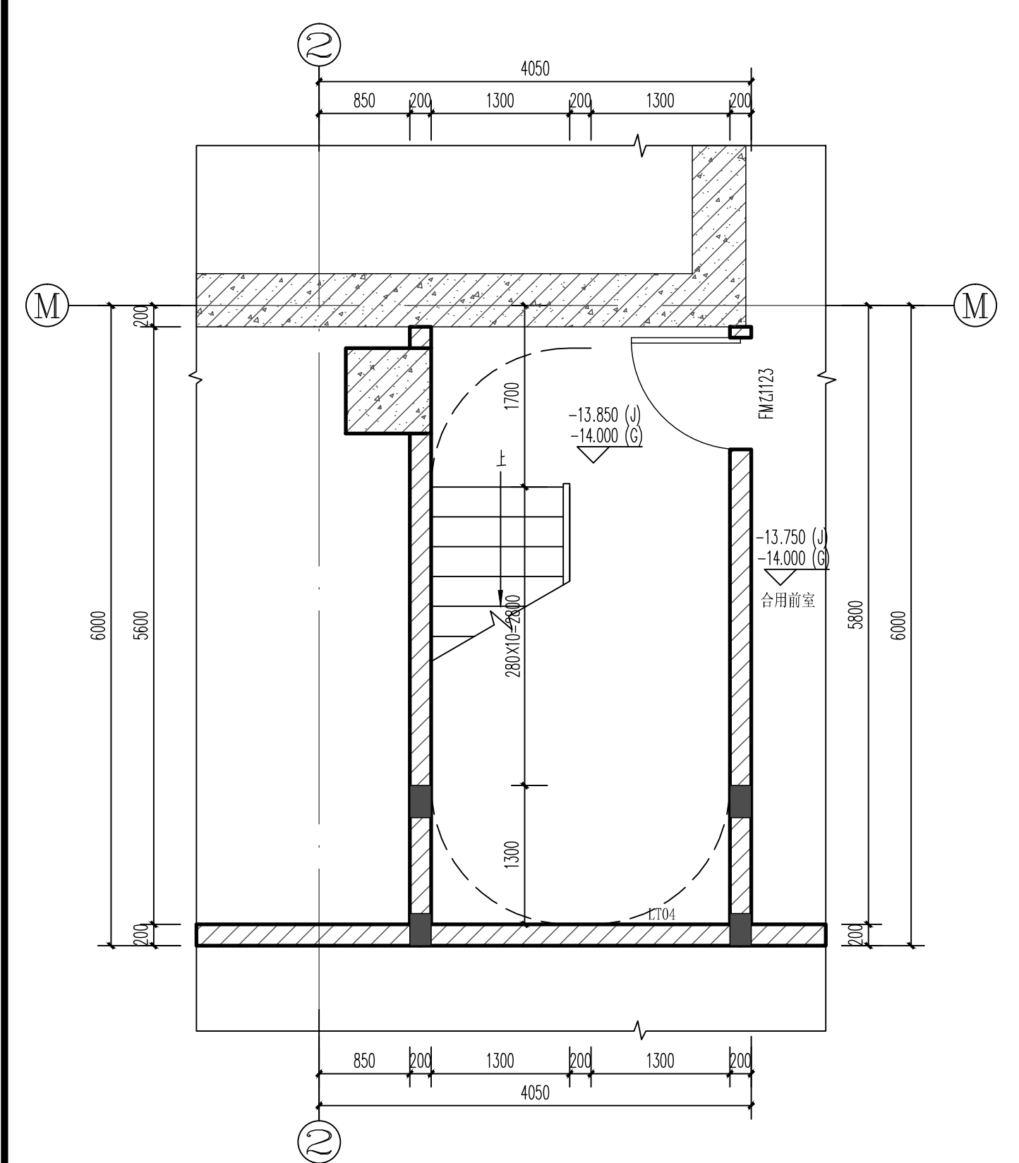
比例 LT04 地下三层平面 1:50
